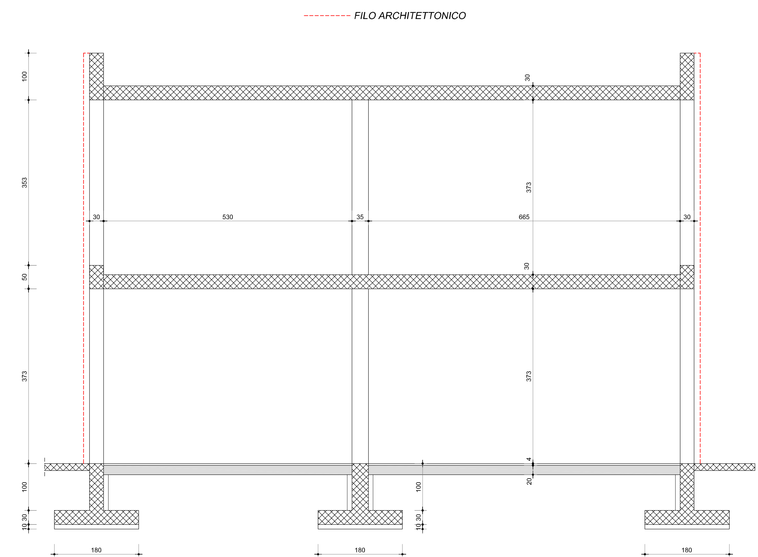
SEZIONE VERTICALE STRUTTURALE X-X rapp. 1:50
