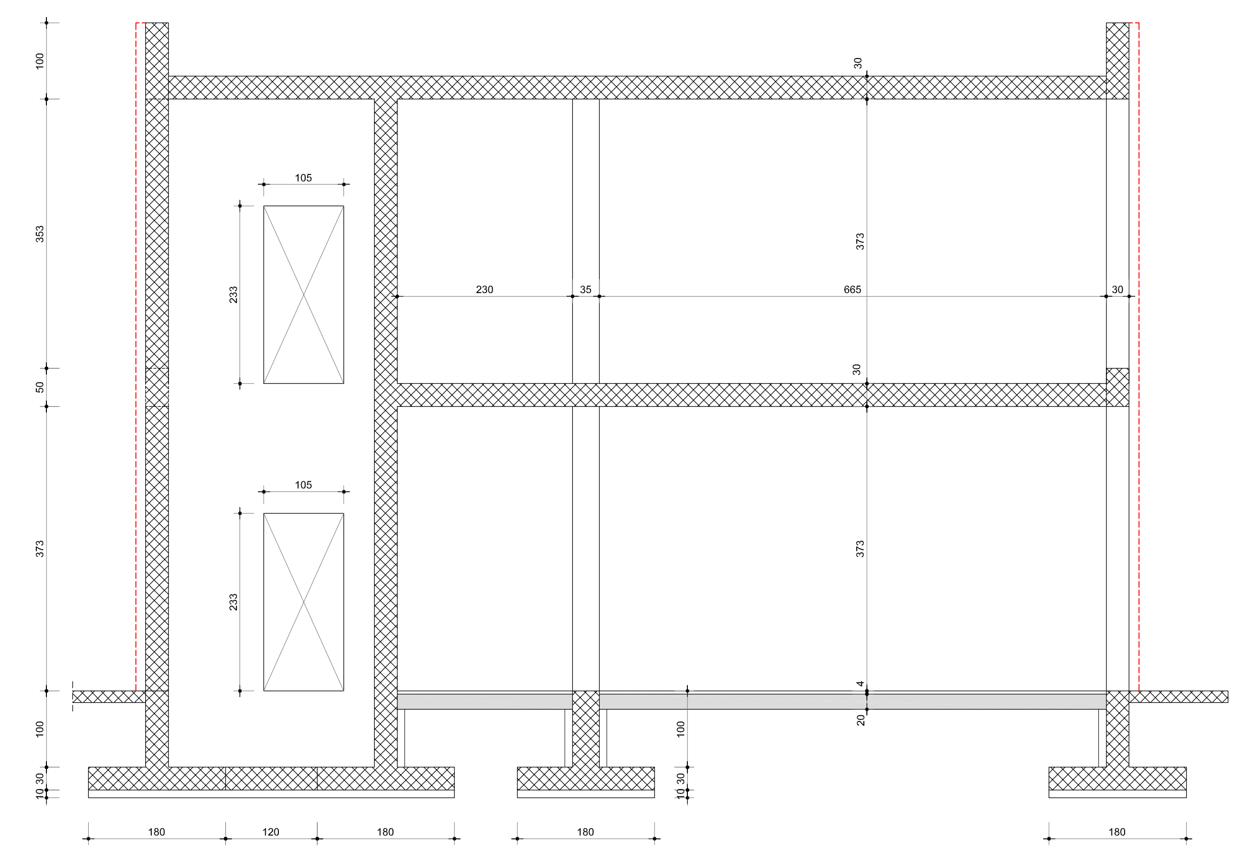
SEZIONE VERTICALE STRUTTURALE Y-Y rapp. 1:50
