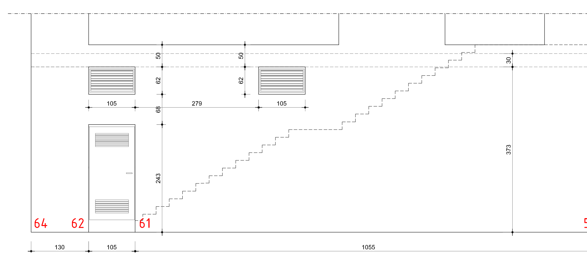
FOROMETRIE SOTTOSOLAIO SETTI 64-62-61-50 rapp. 1:50
