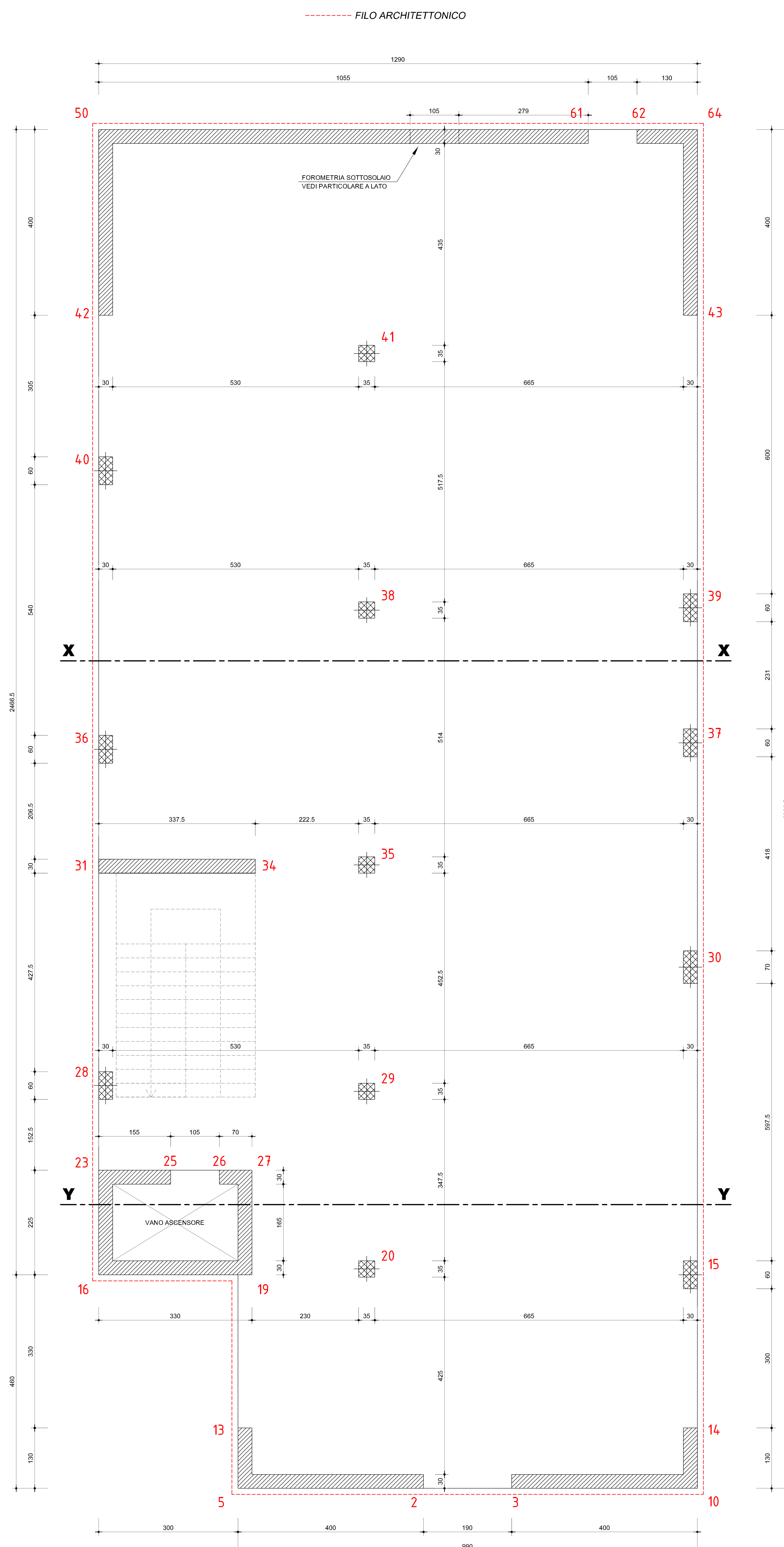
PIANTA DI RIFERIMENTO PIANO TERRA rapp. 1:50
